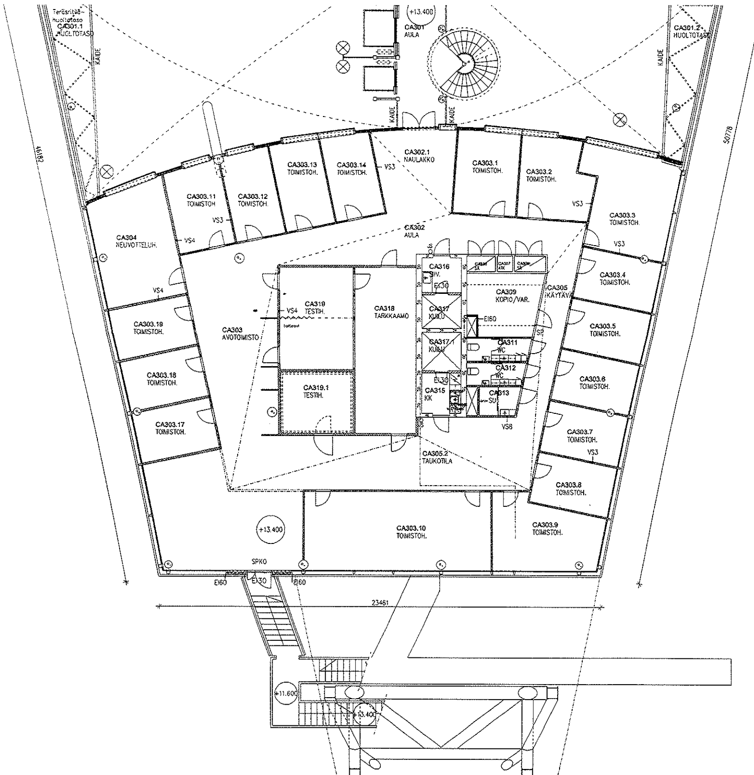
HTC PINTA Helsinki Tammasaarenkatu 3 3.kerros 598,5m 2 n. 1:200 (A4)
